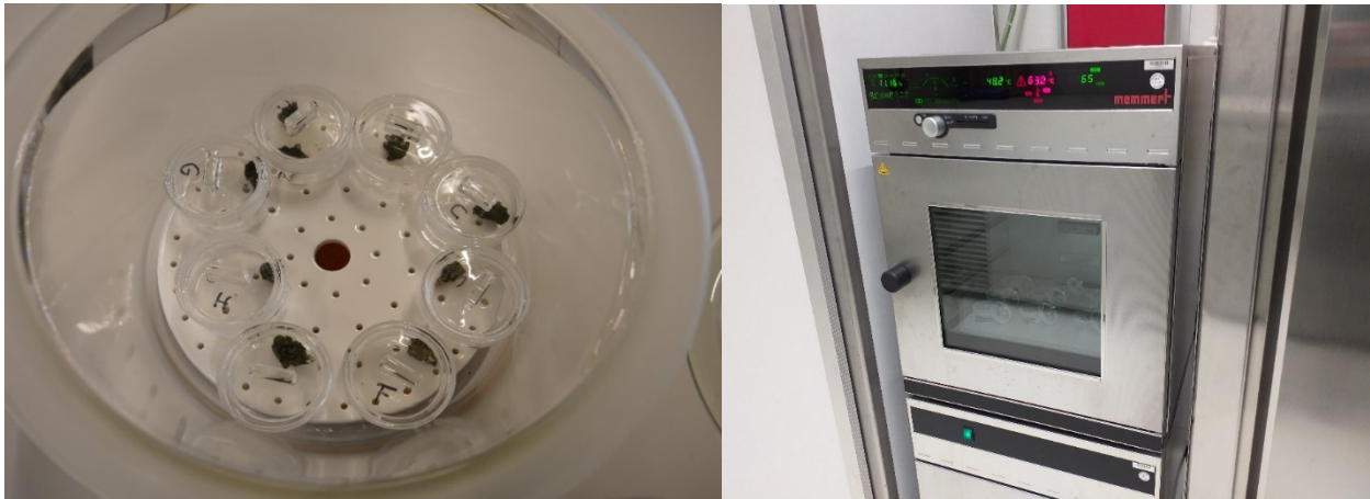
Figuur 7 Mestmonsters in weegpotten (links); drogen van mestmonsters onder vacuüm (< 2.5 kPa) bij 60^{\circ} \pm 3^{\circ}\text{C} (rechts).
